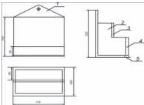
Расми 4. Нақшаи қуттӣ барои бўрмонӣ
