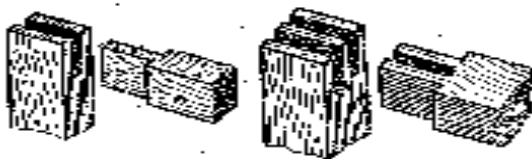
Расми 24. Пайвастагиҳои комакии чузбӣёт: а – яккомакӣ; б – дукомакӣ
