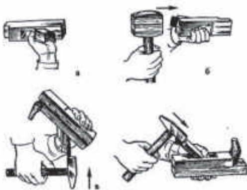
Расми 22. Тайёр намудани ранда ба кор
