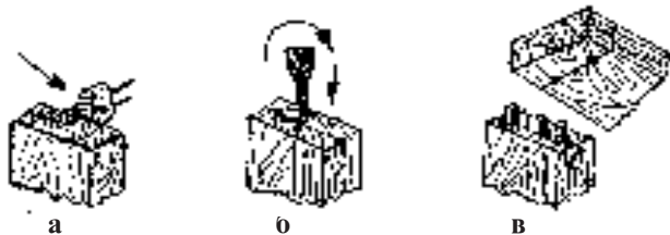
Расми 34. Пайдарпайӣ ва ҷобачокунии чузъиёт бо шкант: а – нишонагузори паҳлу; б – пармакунии сӯроҳӣ ба паҳлу; в – нишонагузорӣ, пармакунии сӯроҳӣ ва пайвасткунӣ
