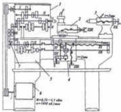
Расми 42. Нақшаи кинематикии дастгоҳи ҳарротии рахпечбур – ТВ-6
