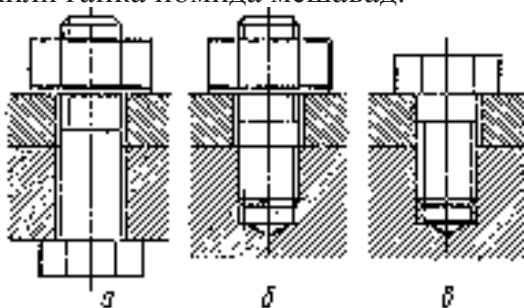
Расми 53. Пайвасти болту гайка, санчок ва винт
