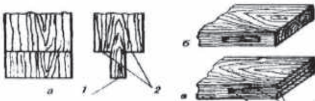
Расми 25. Унсурҳои пайвастагиҳои комакӣ: а – комак; б – лона; в – сӯроҳӣ; 1 – паҳлуи комак; 2 – китфҳо; 3 – рӯяҳо; 4 – таги сӯроҳӣ.
