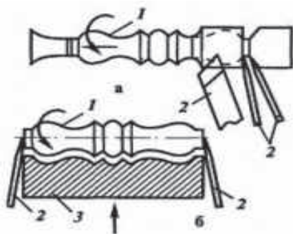
Расми 7. Харротии сатҳҳои муқарнас:
