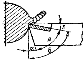
Расми 44. Сохти сарак ё нӯги теғи харротӣ
