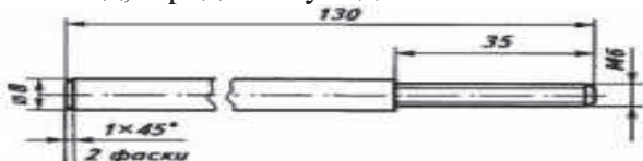
Расми 39. Дастаи қапандаи рахпечбароранда
