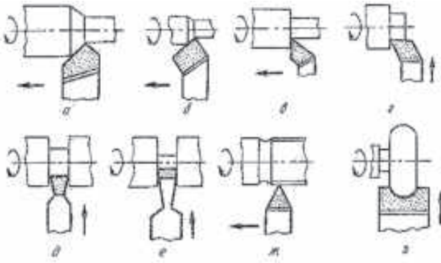
Расми 45. Намудҳои теғи коркарди харротӣ
