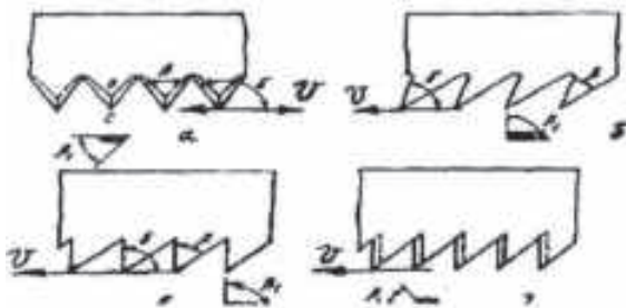
Расми 17. Шакли дандонаҳои арра:
