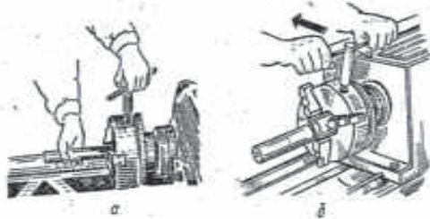
Расми 46. Шинондан ва маҳкам кардани масолеҳ
