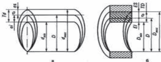
Расми 23. Тамоилӣ ва ҳадди тағйироти андозаҳои чузъиёт
