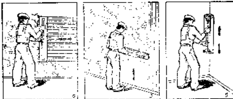
Расми 63. Ҳамвор кардани қабати лойи андова (раствор) дар сатҳи девор:
