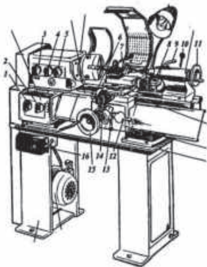
Расми 41. Намуди умумии дастгоҳи ҳарротии рахпечбур – ТВ-6
