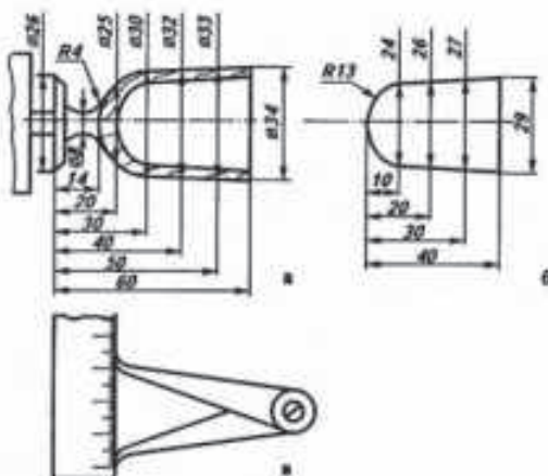
Расми 13. Маснуоти бадеӣ ва асбоб барои назорати андозаҳои дарунӣ: а – нақшаи маснуот; б – қолиб; в – асбоб барои чен кардани қисми дохилӣ бо чадвал
