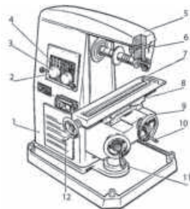
Расми 51. Дастгоҳи уфукӣ-фрезерии тамғаи НГФ-110 Ш4
