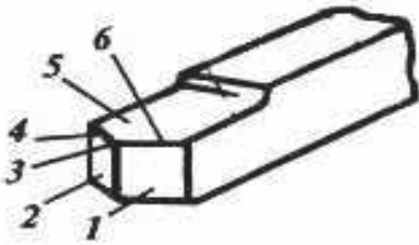
Расми 43. Кунҷҳои буриши теғи харротӣ
