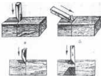
Расми 30. Пайдарпайии буридани сӯроҳӣ: а – буридани кундалангии тағи сӯроҳӣ; б – буридани моилӣ; в – буридани чуқур; г – буридани тарафи муқобил
