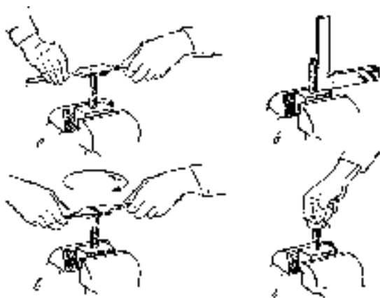
Расми 60. Калид ва рахпечи метрикии дохилӣ бо рахпечбарор
