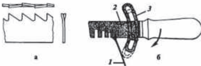
Расми 20. Танзими дандонаҳо: а – бо навбат қатшавии дандонаҳои арра ҳангоми тезкунии; б – танзимкунада: 1 – тасмаи арра, 2 – танзимкунада; 3 – тақя
