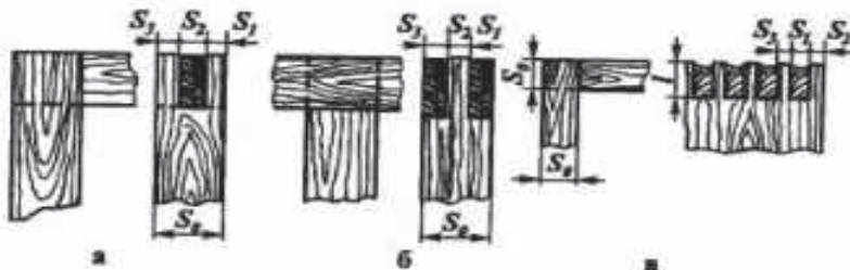
Расми 26. Намудҳои пайвастагиҳои комакӣ: а – охирӣ; б – тамғагӣ; в – қуттигӣ: S_0 – ғафсӣ, S_1 ва S_3 – ғафсии гӯшаҳо, S_2 – ғафсии комак, l – дарозии комак
