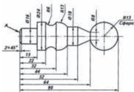
Расми 10. Нақшаи ҷузыёти харротии мукарнасӣ
