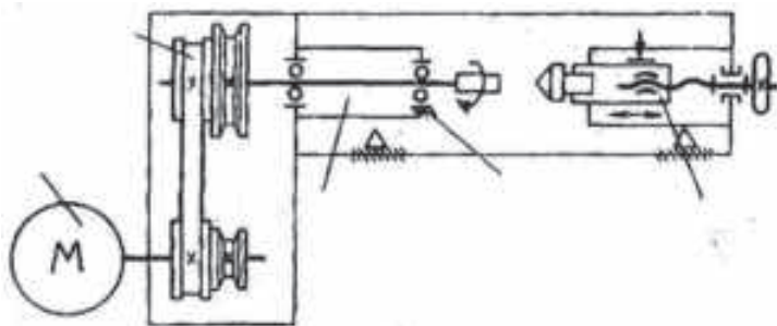
Расми 5. Нақшаи кинематикии дастгоҳи ҳарротии СТД-120 М
