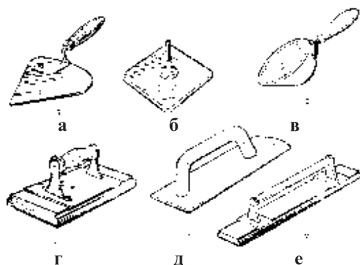
Расми 62. Афзорҳо барои иҷрои корҳои андовакунӣ
