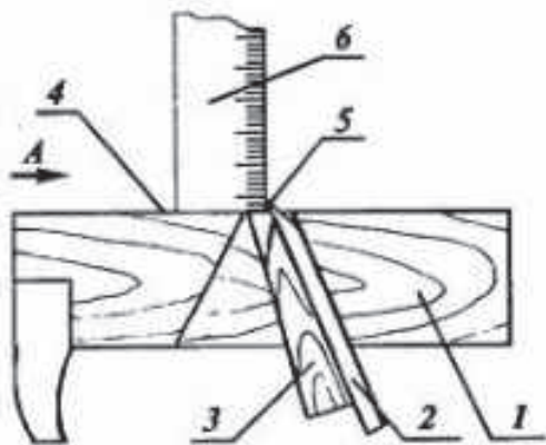
Расми 21. Танзими ранда
