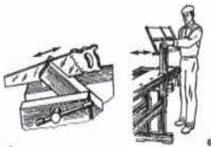
Расми 28. Усулҳои барқақ буридани пайвастиҳои комакӣ:
